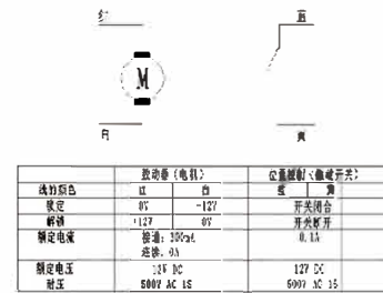
控制接线 Control Wiring
